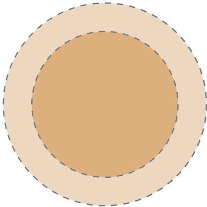
עיגול
