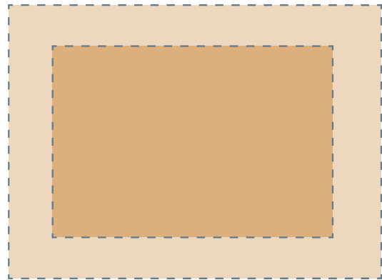
מלבן
