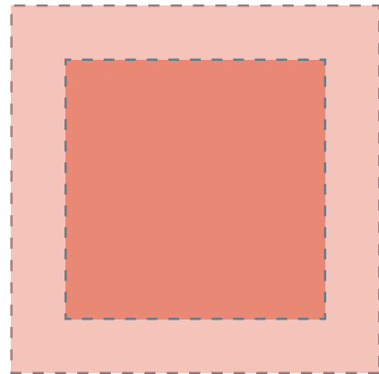
ריבוע
