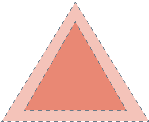
משולש
