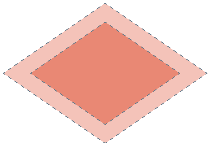
יהלום
