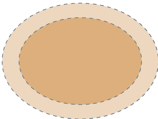
אליפסה
